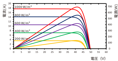
RSM132-8-690BHDG 異なる照射量下でのI-Vカーブ
