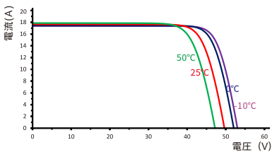
異なる温度下でのI-Vカーブ (AM1.5, 1000W/m²)
